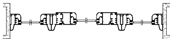
Corte Horizontal
